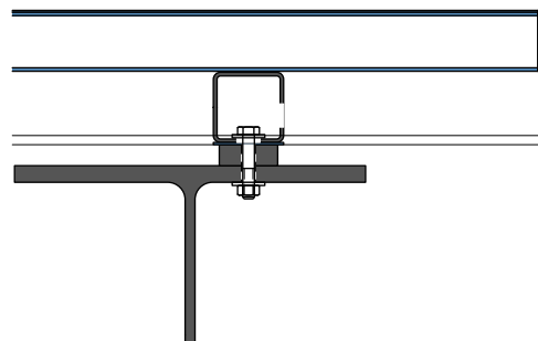
Vertikalschnitt
