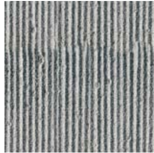
rorschacher_sandstein_sch
