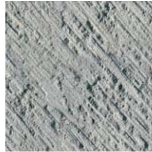
rorschacher_sandstein_gcb
